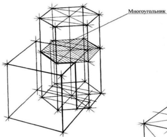
Врезка куба и шестигранной призмы
