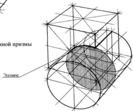
Врезка куба и цилиндра
