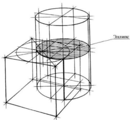
Врезка куба и цилиндра
